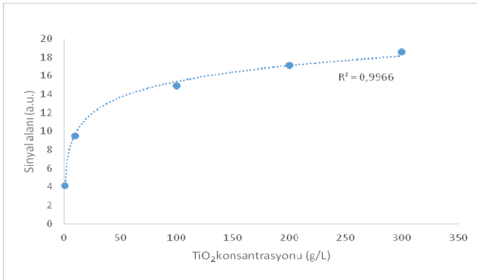
Şekil 9. DMPO çözeltisi ile UV ışık altında etkileşime sokulan 1, 10, 100, 200 ve 300 g/L \text{TiO}_2 ile elde edilen ESR sinyallerinin alanları
