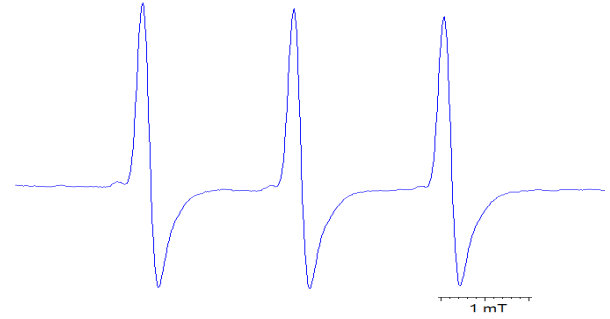
Şekil 10. 30 \mu\text{M} TEMPO çözeltisinin ESR spektrumu
