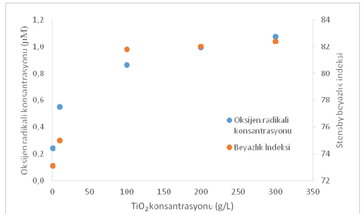
Şekil 12. 1, 10, 100, 200 ve 300 g/L \text{TiO}_2 varlığında UV ışık altında salınan oksijen radikali konsantrasyonları ve aynı konsantrasyonlarda elde edilen beyazlık değerleri
